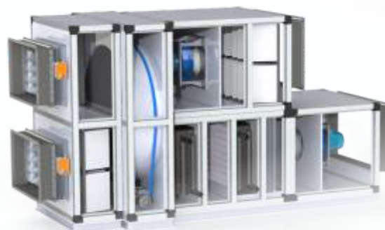
Центральный кондиционер приточно-вытяжной с рекуператором
